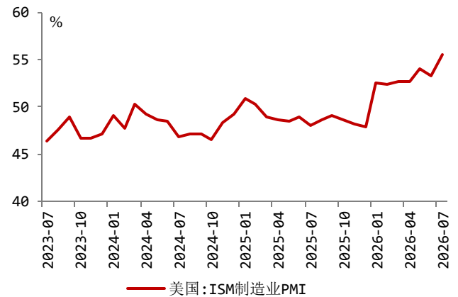
图 4：美国制造业景气指数走势
